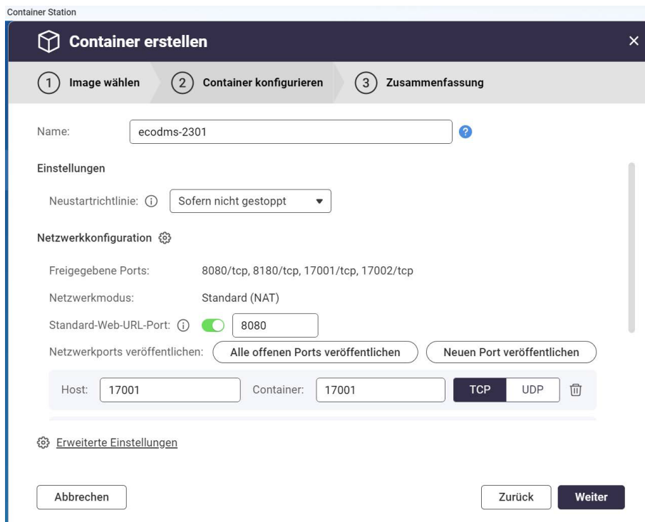
Abb. (ähnlich) 4.19: QNAP - Container Name vergeben
