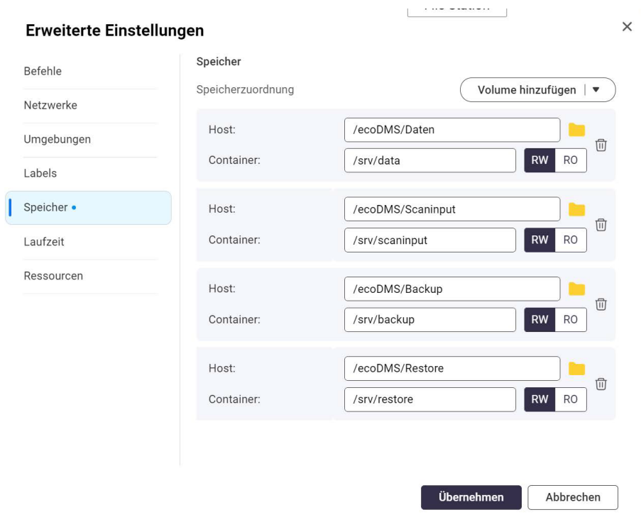
Abb. (ähnlich) 4.21: QNAP - Erweiterte Einstellungen - Speicher
