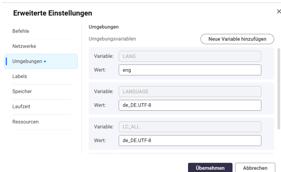
Abb. (ähnlich) 4.22: QNAP - Erweiterte Container Einstellungen - Sprache ändern
